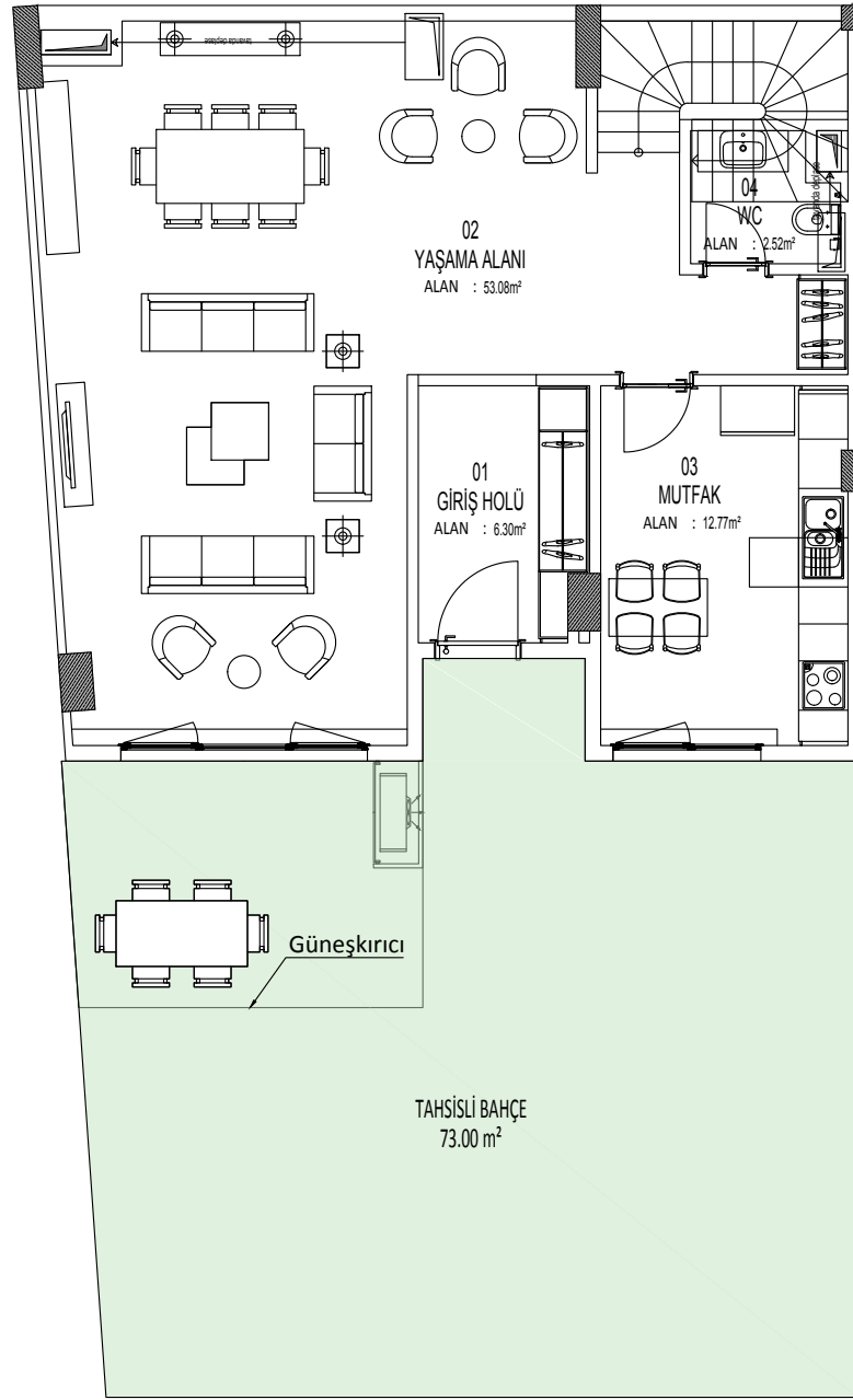
ZEMİN KAT
