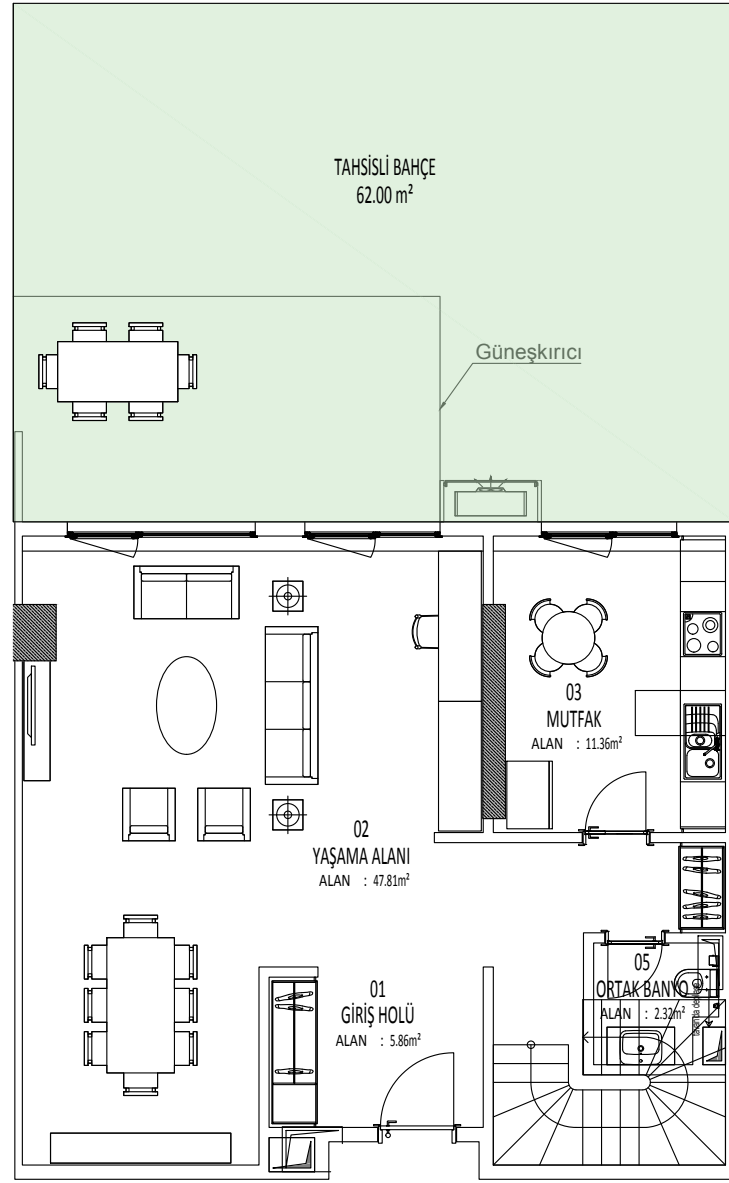
-1.BAĞÇE KATI
