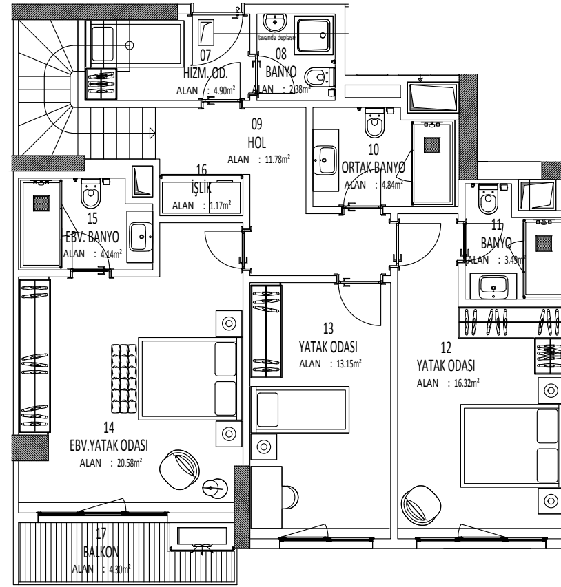
1. KAT
