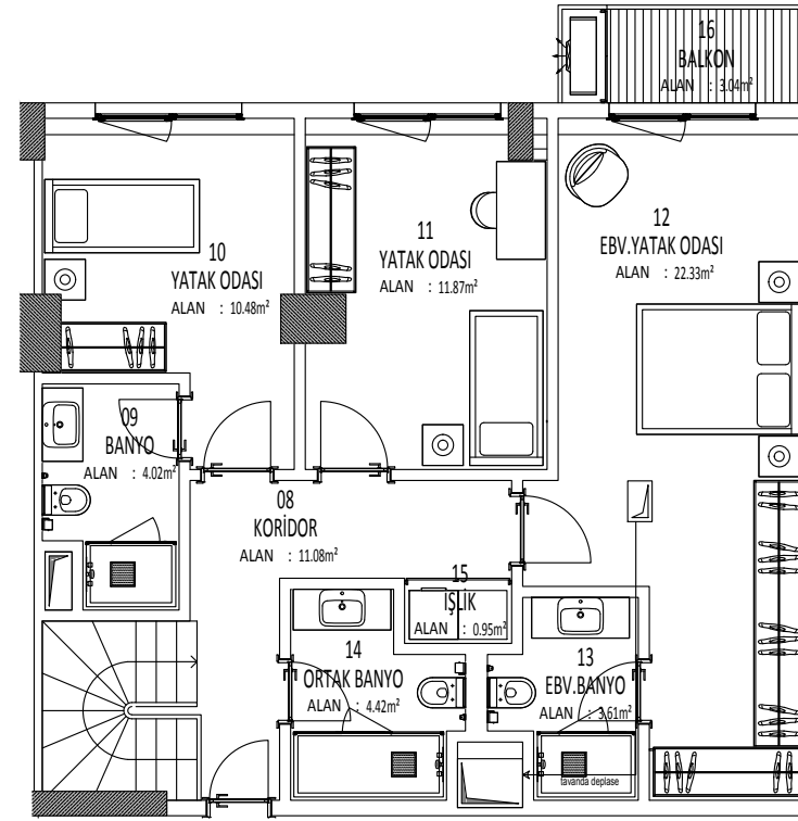
ZEMİN KAT
