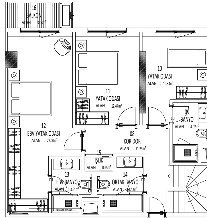
ZEMİN KAT
