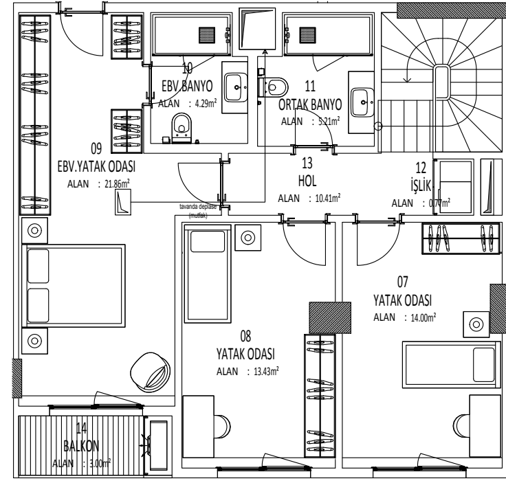
1. KAT
