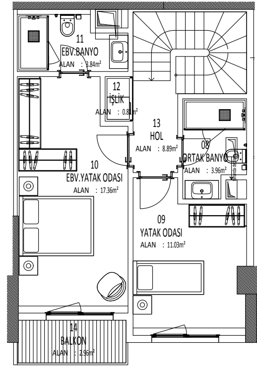
1. KAT
