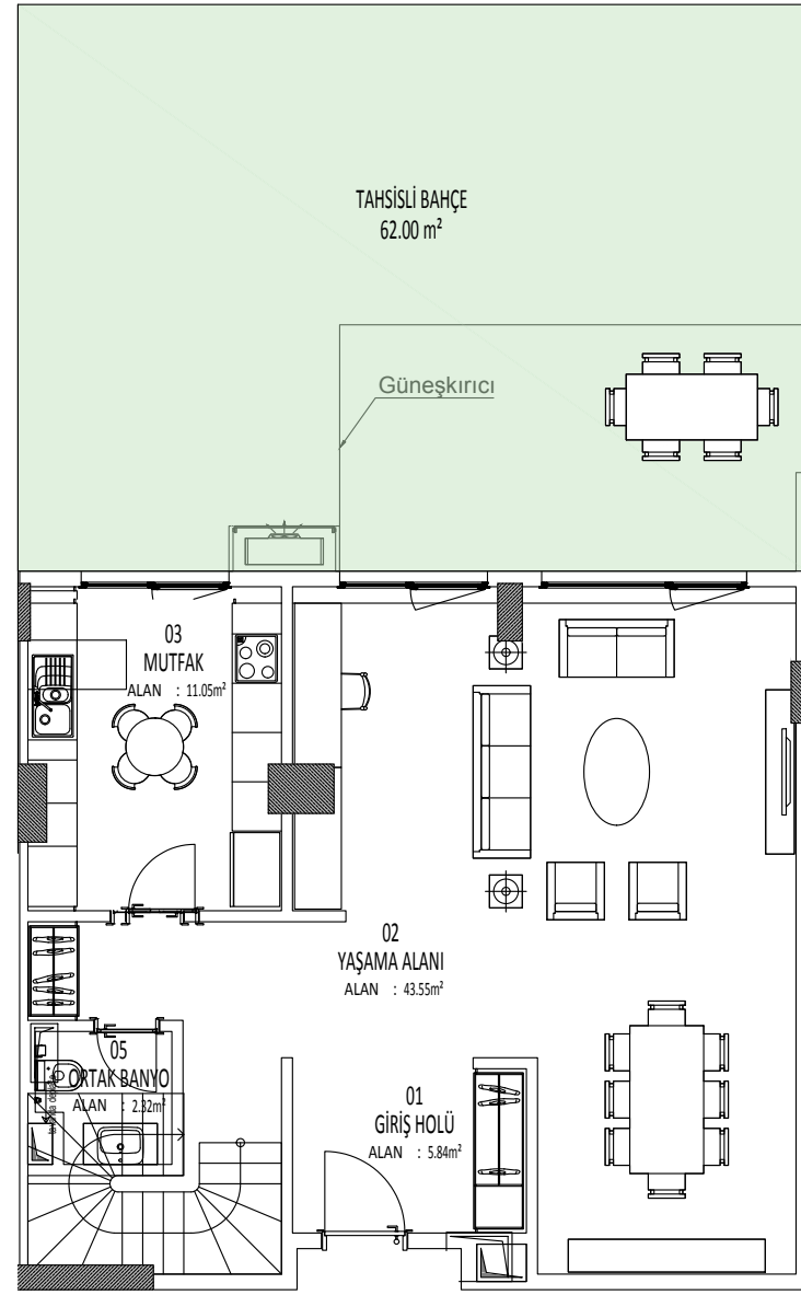
-1.BAĞÇE KATI
