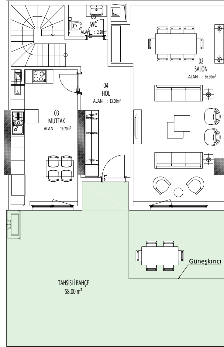
ZEMİN KAT
