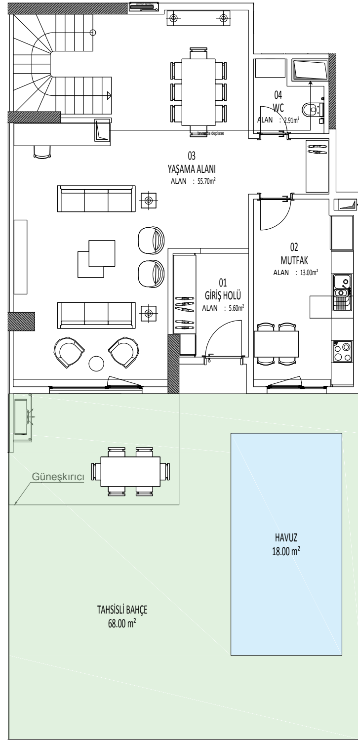
ZEMİN KAT
